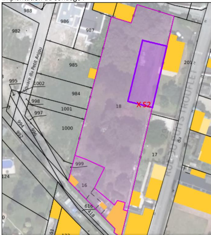
Figure 2 : plan d'implantation du sondage de sol
