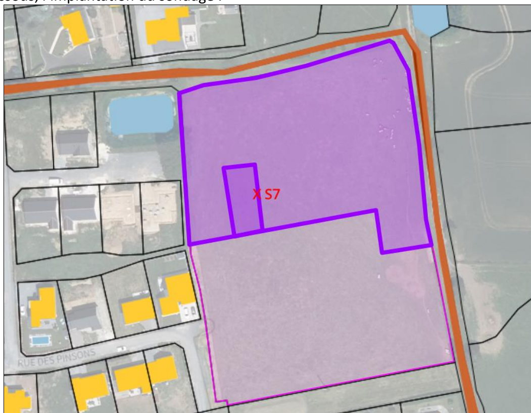
Figure 2 : plan d'implantation du sondage de sol
