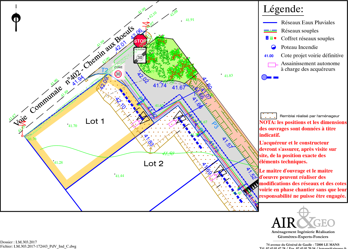
EXTRAIT DE PLANS VRD - Echelle: 1/500
