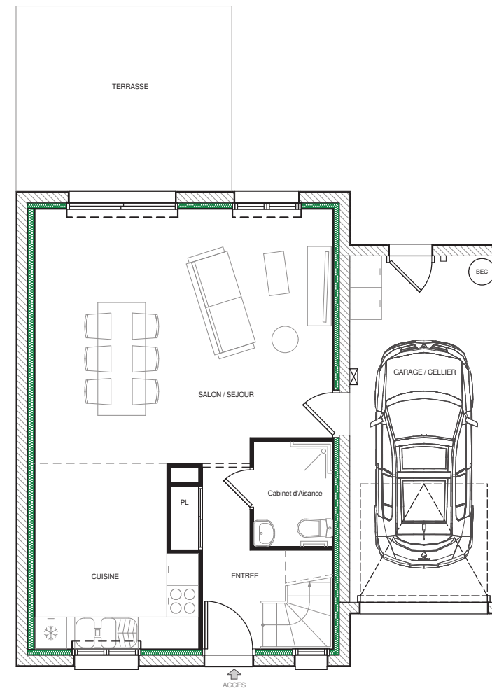
NIVEAU REZ-DE-CHAUSSEE
