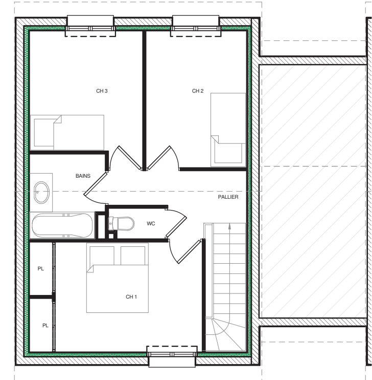
NIVEAU ETAGE
