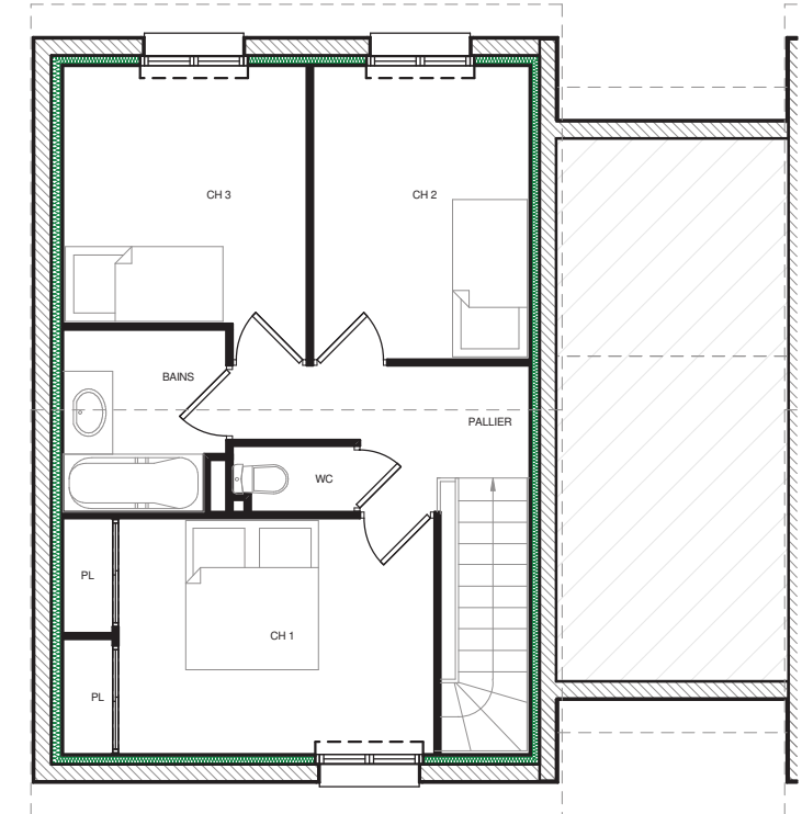
NIVEAU ETAGE
