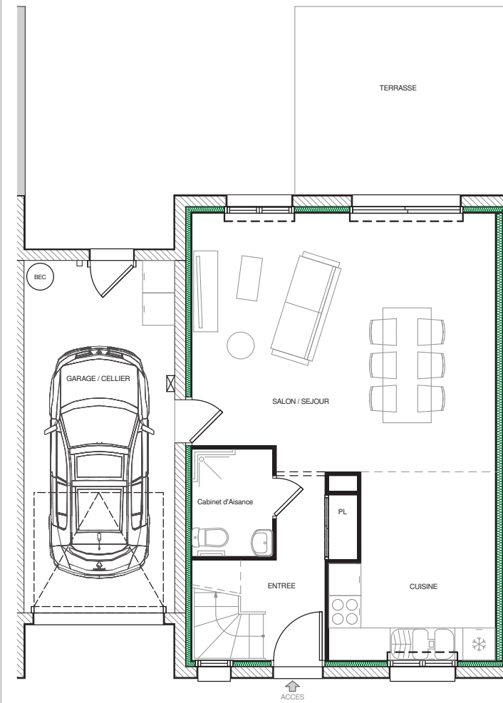
NIVEAU REZ-DE-CHAUSSEE
