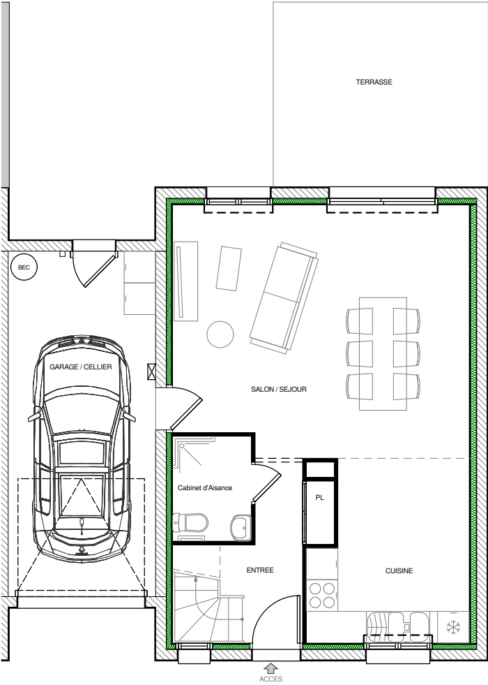
NIVEAU REZ-DE-CHAUSSEE
