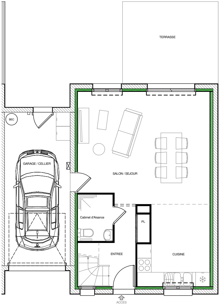
NIVEAU REZ-DE-CHAUSSEE
