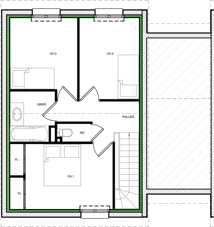
NIVEAU ETAGE
