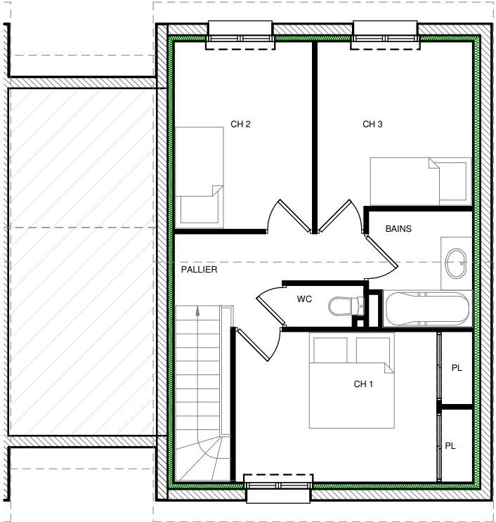
NIVEAU ETAGE
