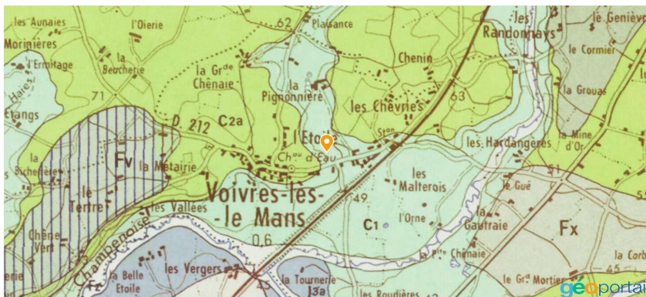
Carte géologique
