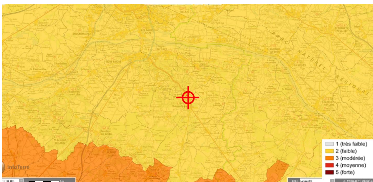
Figure 7 : Cartographie du zonage sismique sur le secteur étudié, échelle 1/100 000 (source BRGM)
