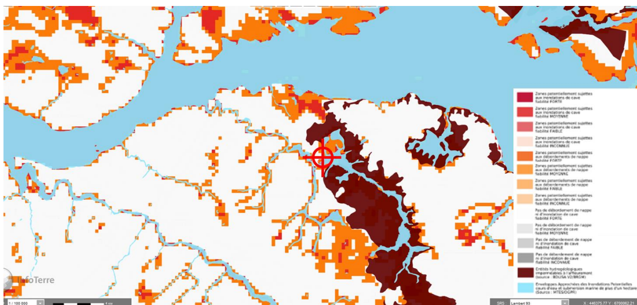
Figure 6 : Cartographie de l'aléa Remontée de nappes sur le secteur étudié, échelle 1/100 000 (source BRGM)
