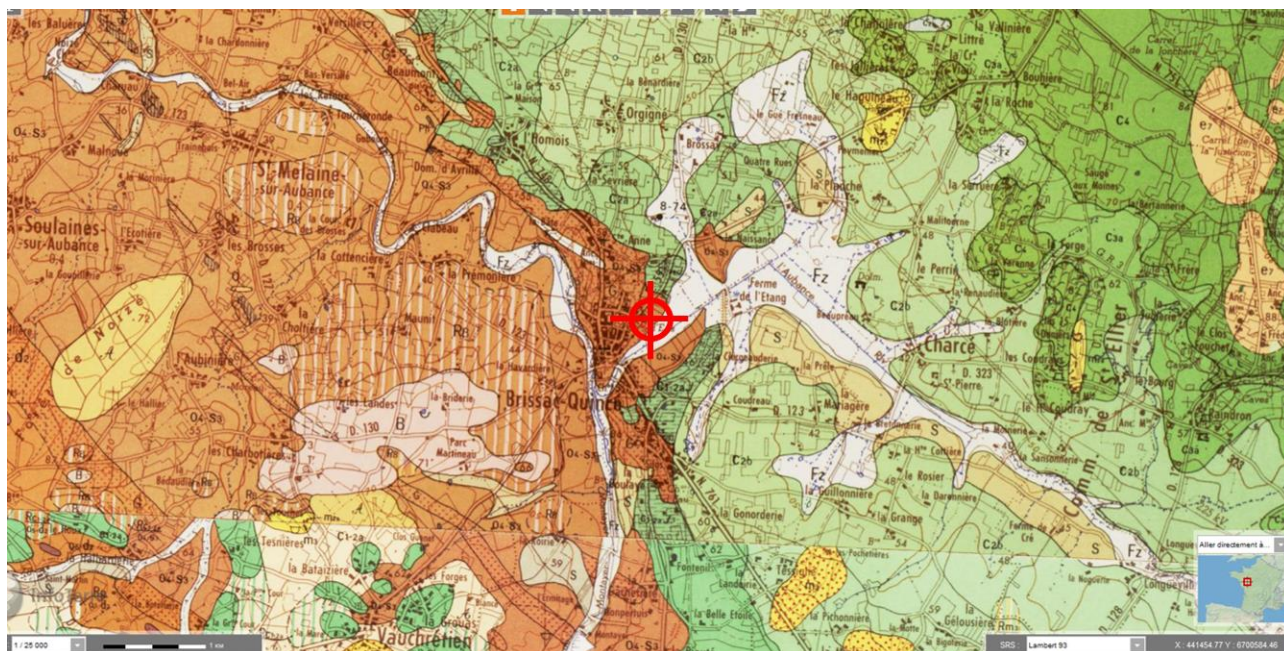
Figure 4 : Extrait de la carte géologique 454, échelle 1/25 000 (source BRGM)
