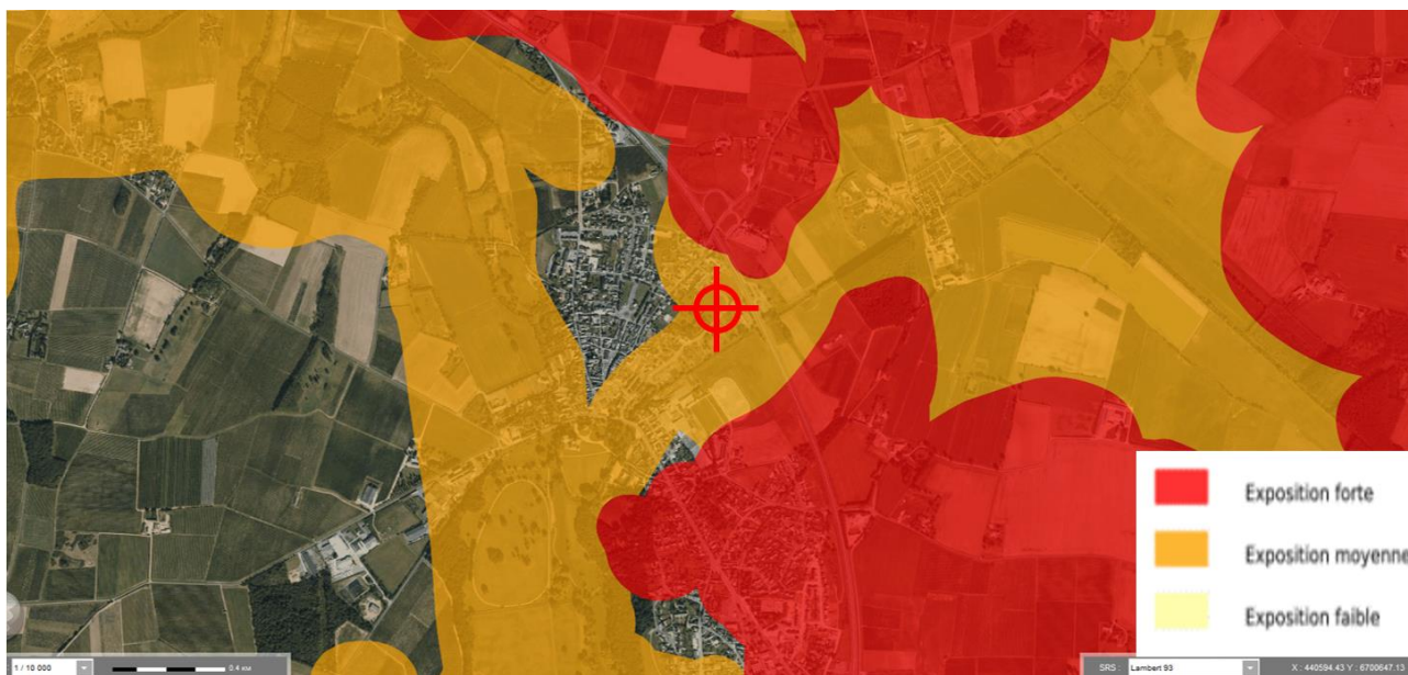
Figure 5 : Cartographie de l'aléa Retrait-Gonflement des Argiles sur le secteur étudié, échelle 1/10 000 (source BRGM)
