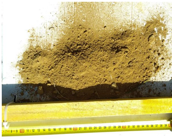
Photographie des prélèvements à la tarière T20 (faciès d'argile d'altération)
