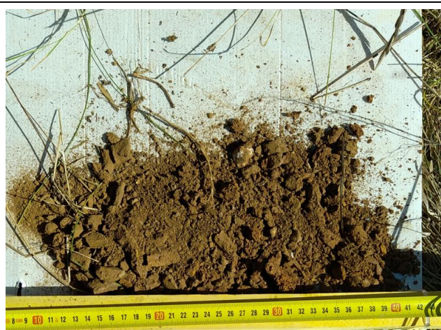
Photographie des prélèvements à la tarière T8 (faciès d'argile d'altération)
