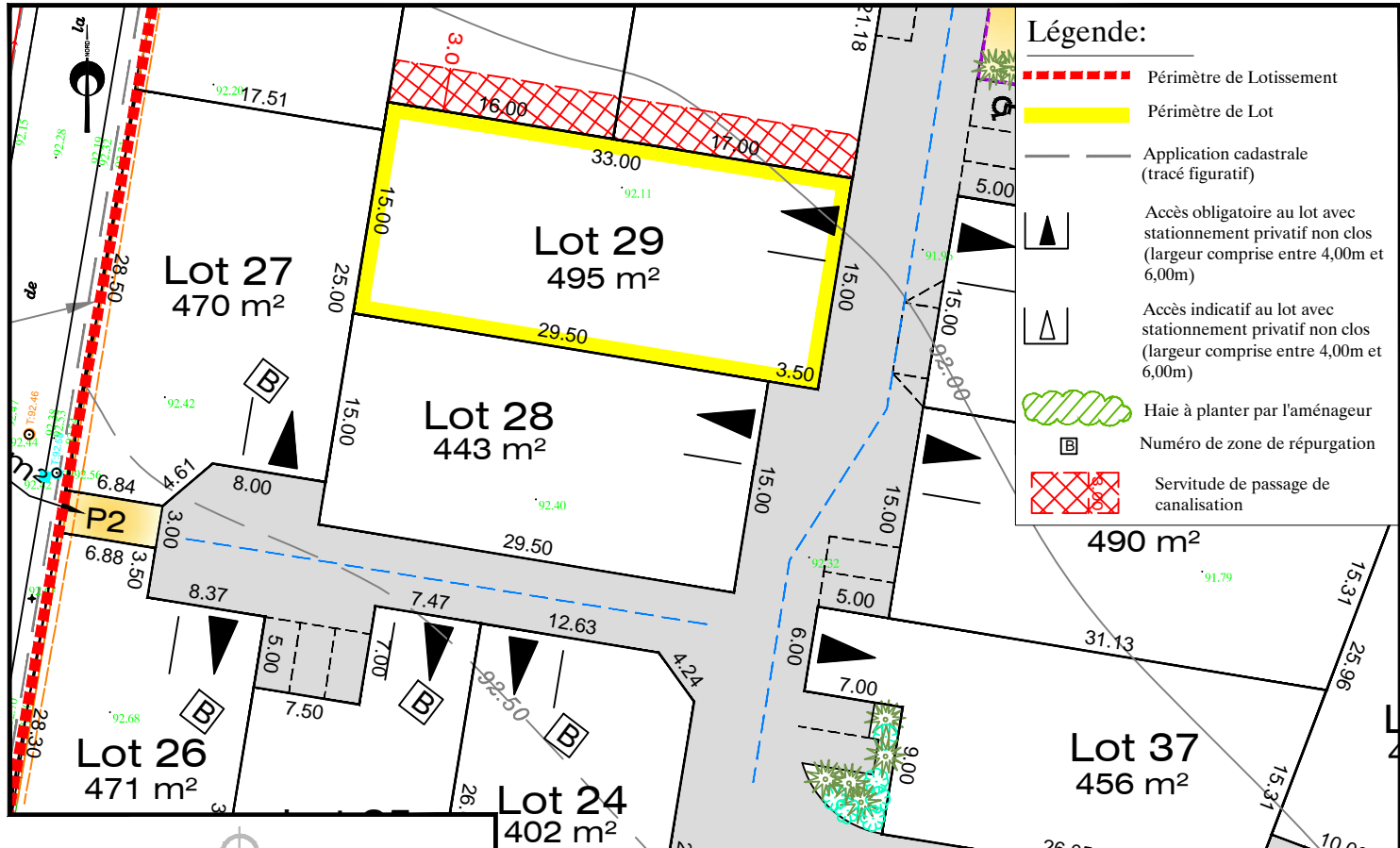
PLAN DE COMPOSITION - Echelle: 1/500
